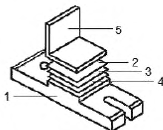
1 – стальная опорная плита; 2 – лента с двойным липким слоем; 3 – образец картона; 4 – лента с двойным липким слоем; 5 – алюминиевое прижимное устройство Рисунок 1– Сформированная проба для испытания образца картона
