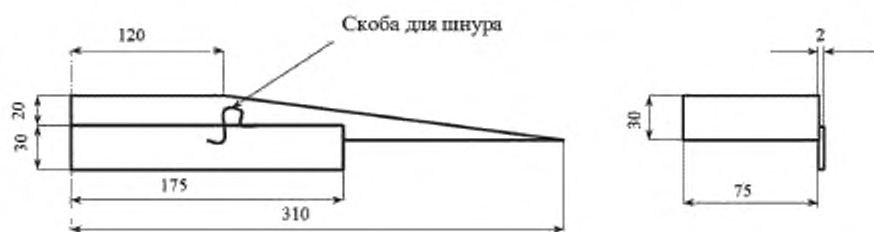
Рисунок А.1 — Клин для возбуждения колебаний обрессоренных частей экипажа
