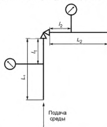
б) Участок стенда для испытания угловой арматуры
