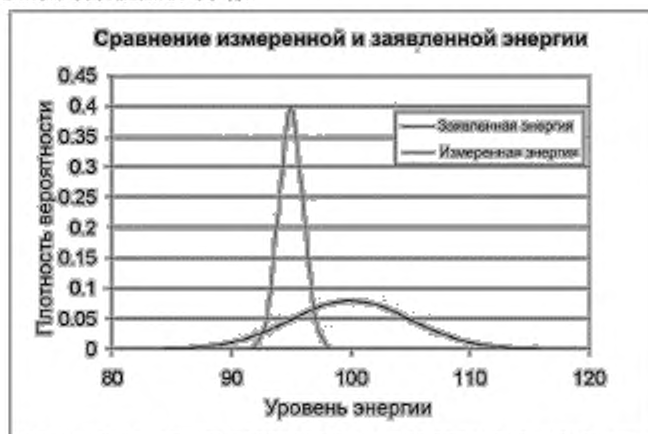
Рисунок 2 – Сравнение измеренной и заявленной энергии
