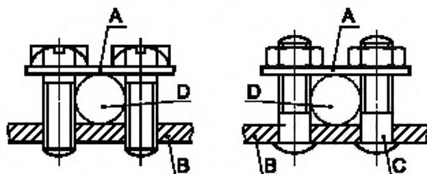
Рисунок 2 — Примеры винтовых и шпильчных зажимов
