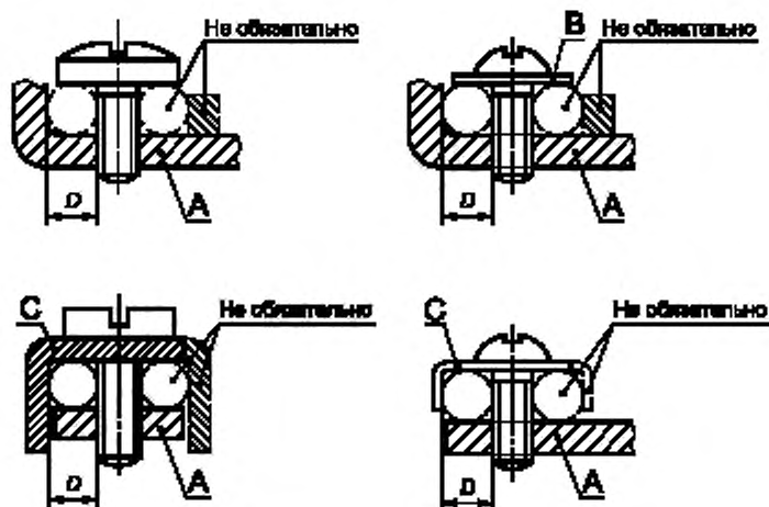
Рисунок 2а — Винтовые зажимы
