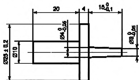
Рисунок 13 — Испытательный стержень
