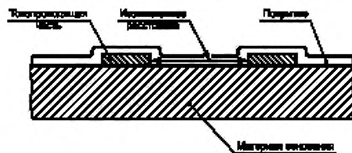
Рисунок Q.1 — Измерение изоляционного расстояния
