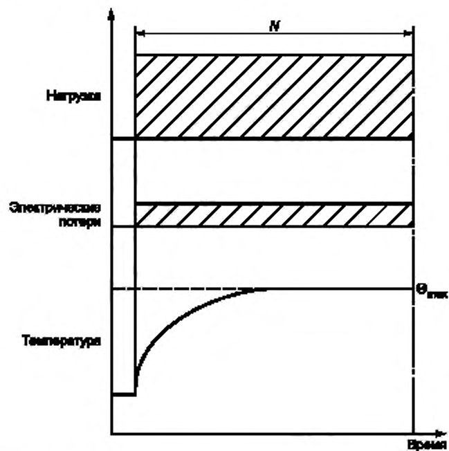
Рисунок 14 — Непрерывный режим работы (тип режима работы S1) (см. 7.1.16.1)
