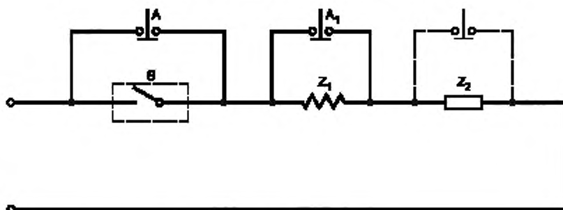
Рисунок 18 — Схема для испытания на нагрев
