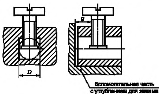
Рисунок 1b — Примеры колонковых зажимов с прижимными пластинами
