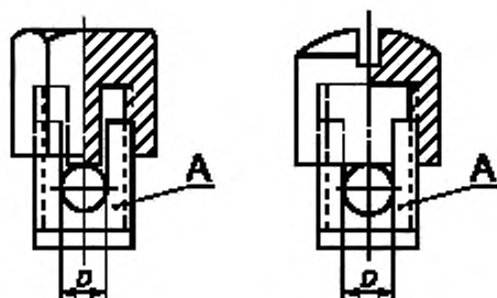
Рисунок 4 — Примеры зажимов под наконечник
