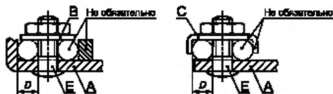
Рисунок 2b — Шпильчные зажимы
