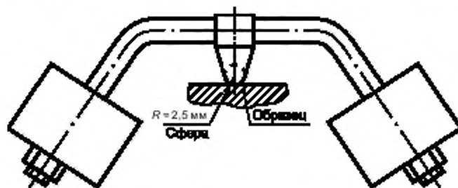
Рисунок 12 — Устройство для вдавления шарика
