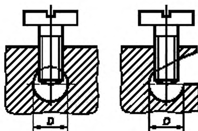
Рисунок 1а — Зажимы без прижимных пластин
