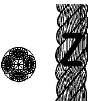
Рисунок 2 – Конфигурация 4-рядного (shroud-laid) каната (тип В)
