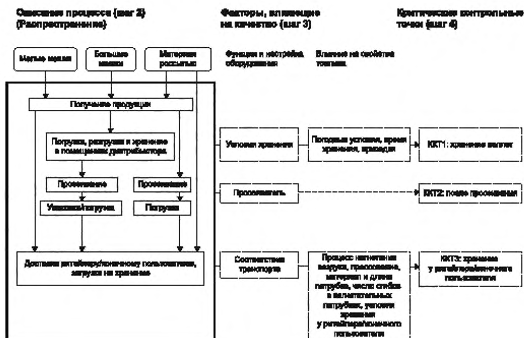
Схема 3 — Пример описания цепочки поставки с факторами, влияющими на качество, и критическими контрольными точками
