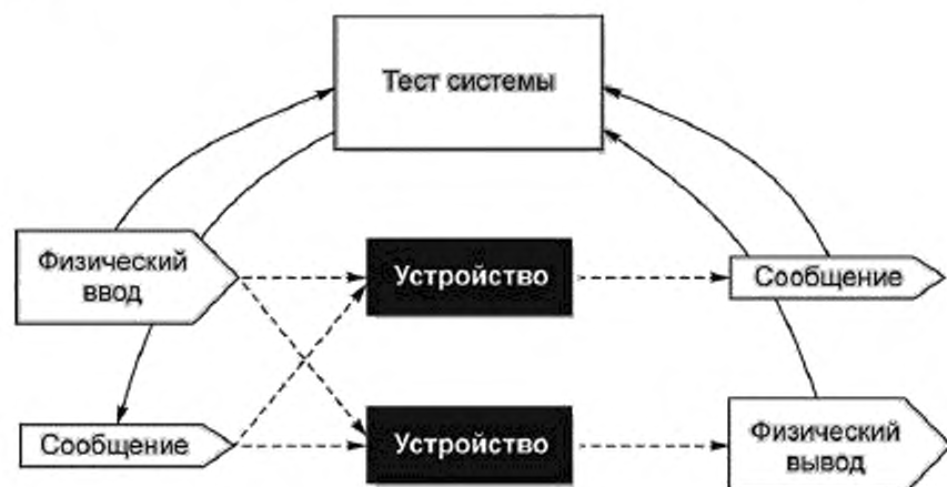
Рисунок 5 — Тестирование производительности (принцип черного квадрата)
