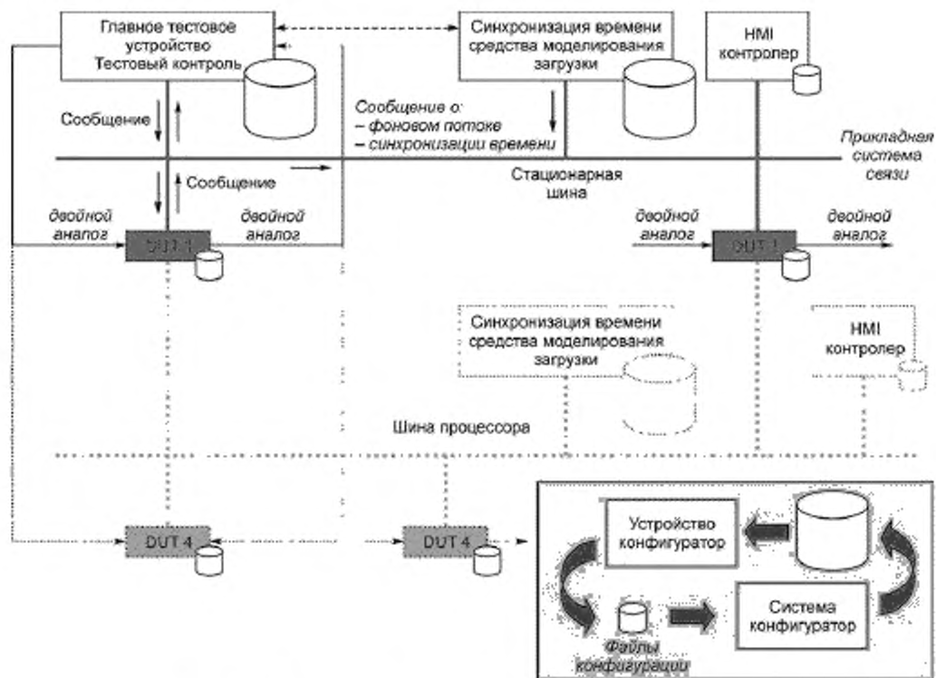
Рисунок 3 — Концептуальная архитектура системы тестирования
