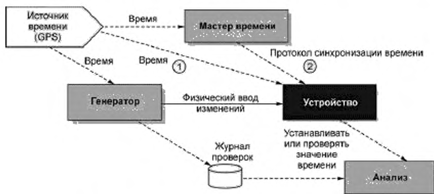
Рисунок 6 — Синхронизация времени и точность проверки установки
