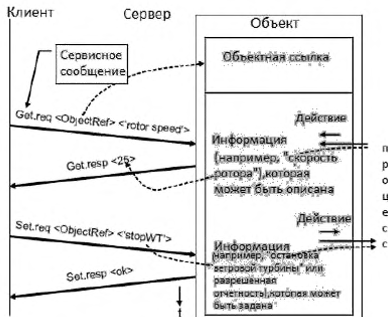
Рисунок В - IEM сервисная модель с примерами
