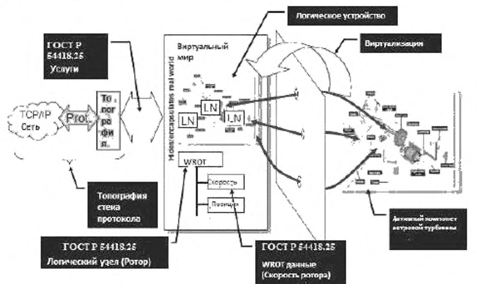
Рисунок 3 – Модельный подход (концептуальный)
