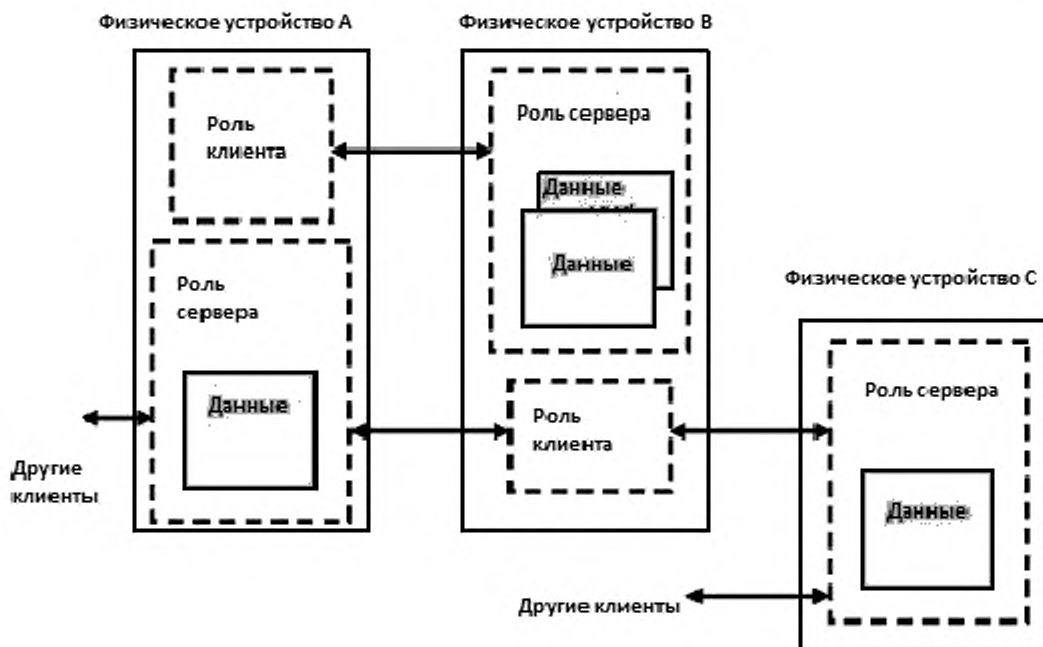
Рисунок 5 – Роль пользователя и сервера
