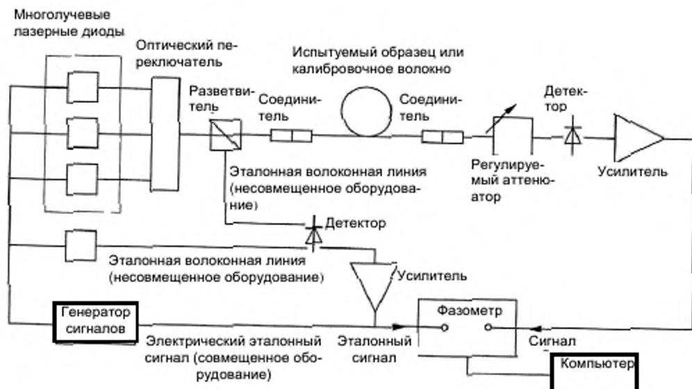
Рисунок А.1 – Комплект оборудования для измерения хроматической дисперсии. Система на основе многолучевого лазера (типовая)
