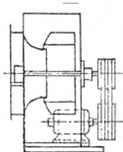
Рисунок 2 – Вентилятор с приводом
