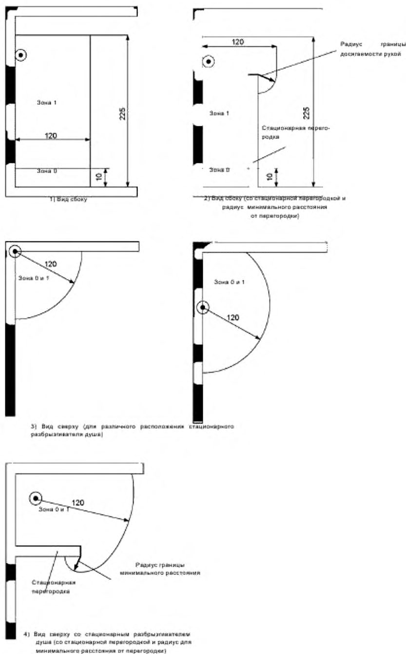
Рисунок 701.2 – Размеры зоны 0 и 1 в помещениях, содержащих душ без поддона
