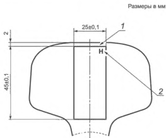
Надрез наносят со стороны верха образца (стрелка 1). верх образца обозначают клеймом «Н» на торце образца (стрелка 2)
