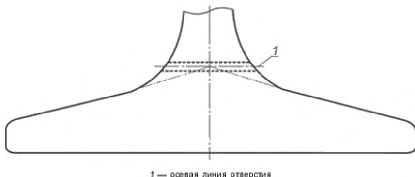
Рисунок К.5 — Расположение отражателя в подошве образца
