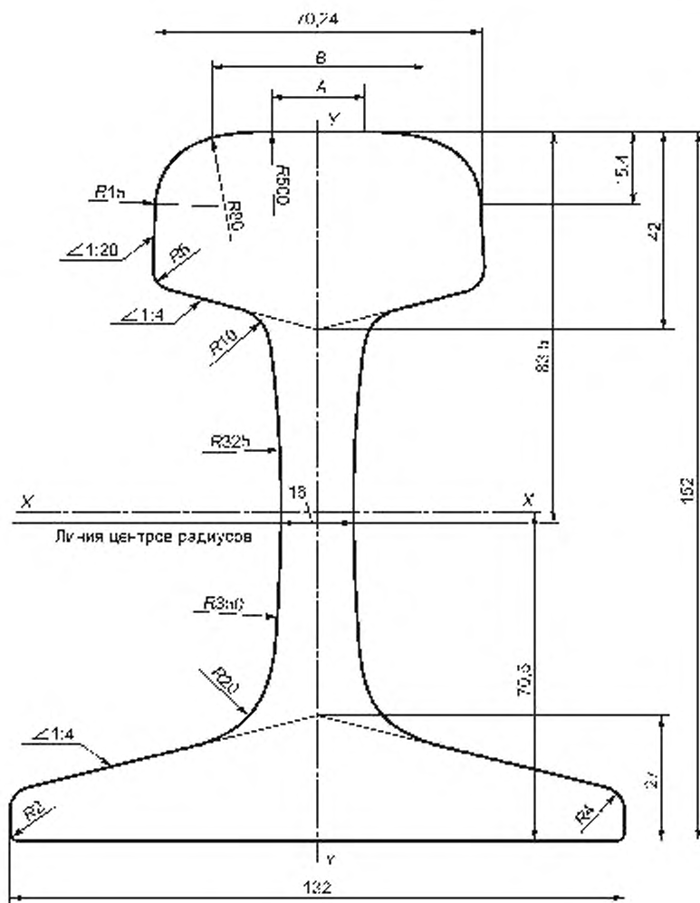
Рисунок Г.1 — Рельс типа P50
