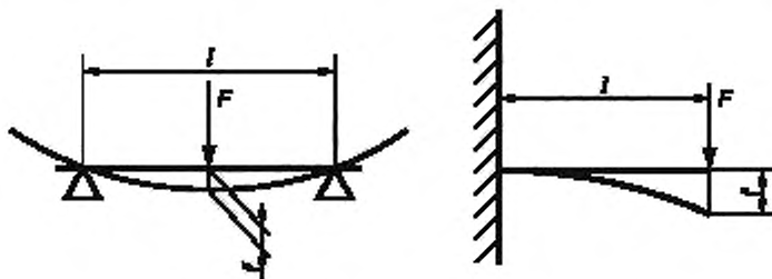
Рисунок 9 — Пример нагружения элементов тренажера
