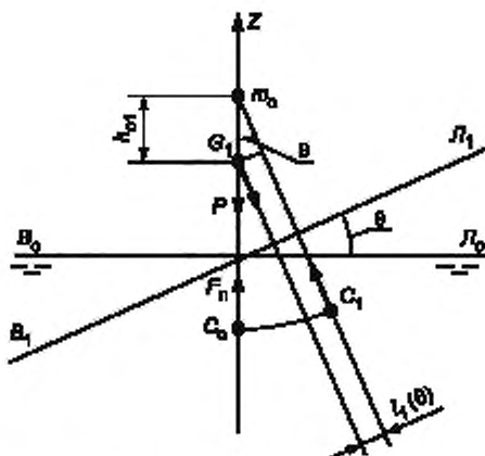
Рисунок К.2 — Плечо статической остойчивости
