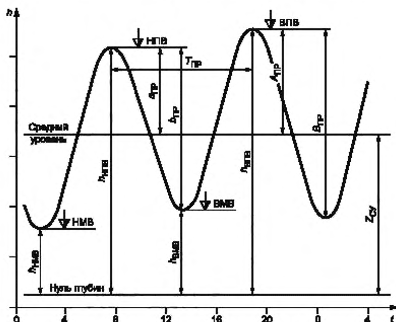
Основные элементы приливных колебаний уровня моря*
