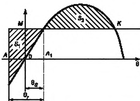
Рисунок 2 — Определение опрокидывающего момента наплавного блока по диаграмме статической остойчивости
