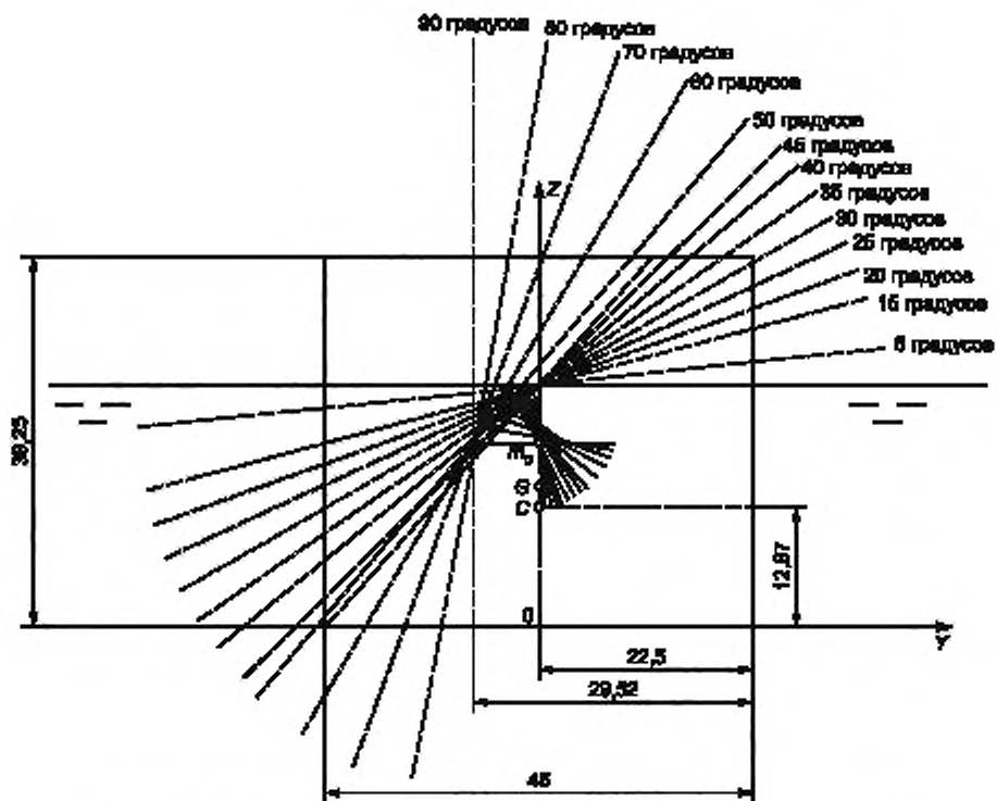
Рисунок К.8 — Положения ватерлиний и соответствующих им перпендикуляров при изменении углов крена от 0^\circ до 90^\circ
