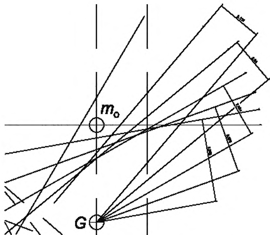
Рисунок К.11 — Измеренные плечи пар сил L(\theta) , при кренах от 0^\circ до 140^\circ
