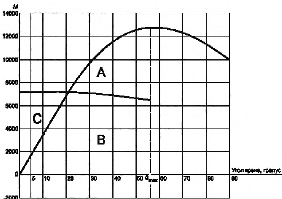
Рисунок 1 — Диаграмма статической устойчивости
