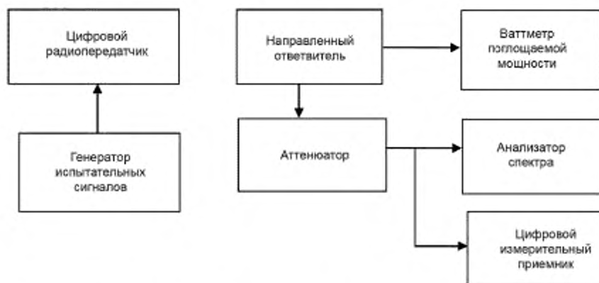
Рисунок 2 — Структурная схема для измерения параметров цифровых радиопередатчиков
