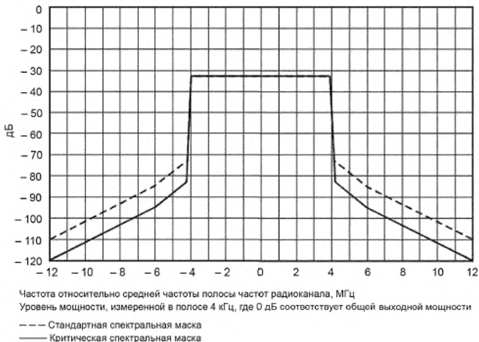
Рисунок 1 — Вид ограничительной маски спектра выходного сигнала радиопередатчика по стандартам DVB T/T2
