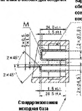
М-М
