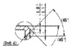
Деталь L
