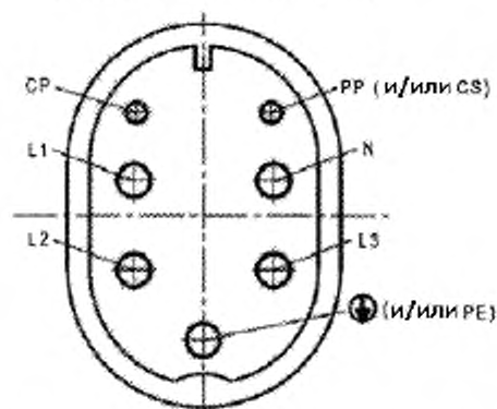
Расположение штырей (вид со стороны штырей)
