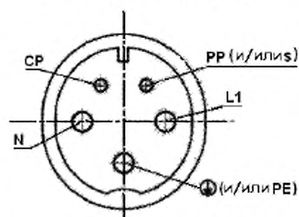
Расположение штырей (вид со стороны штырей)
