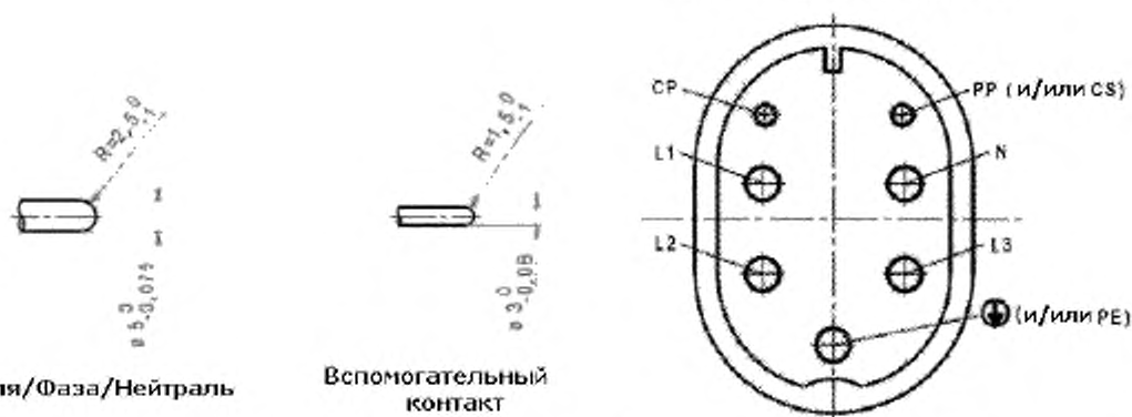
Расположение штырей (вид со стороны штырей)
