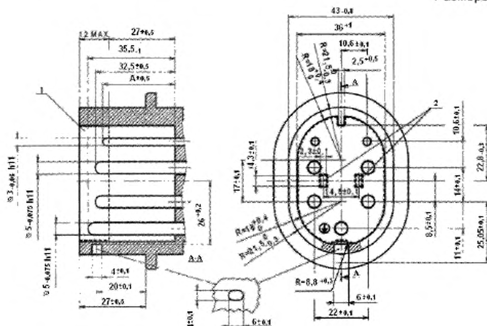
Конец штырей
