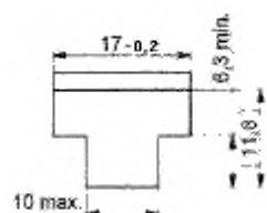
Вид U – показывает максимальные размеры контура защелки
