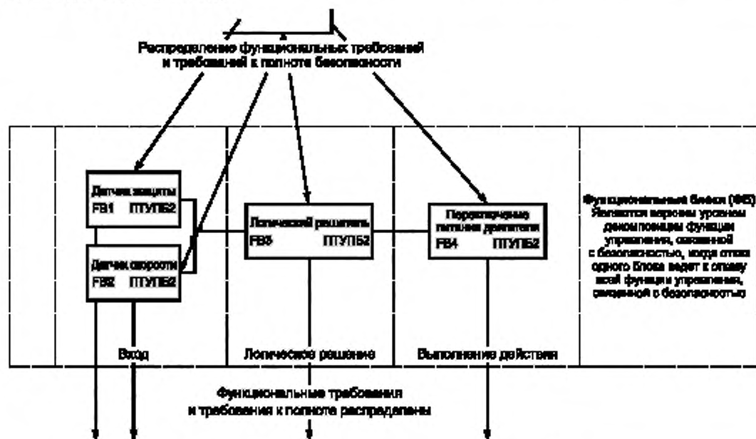
Рисунок В.5 — Начальная концепция архитектуры СБЗСУ
