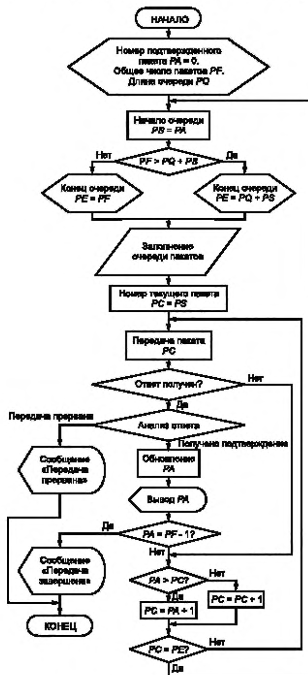
Рисунок 7 — Блок-схема алгоритма процесса передачи данных файла
