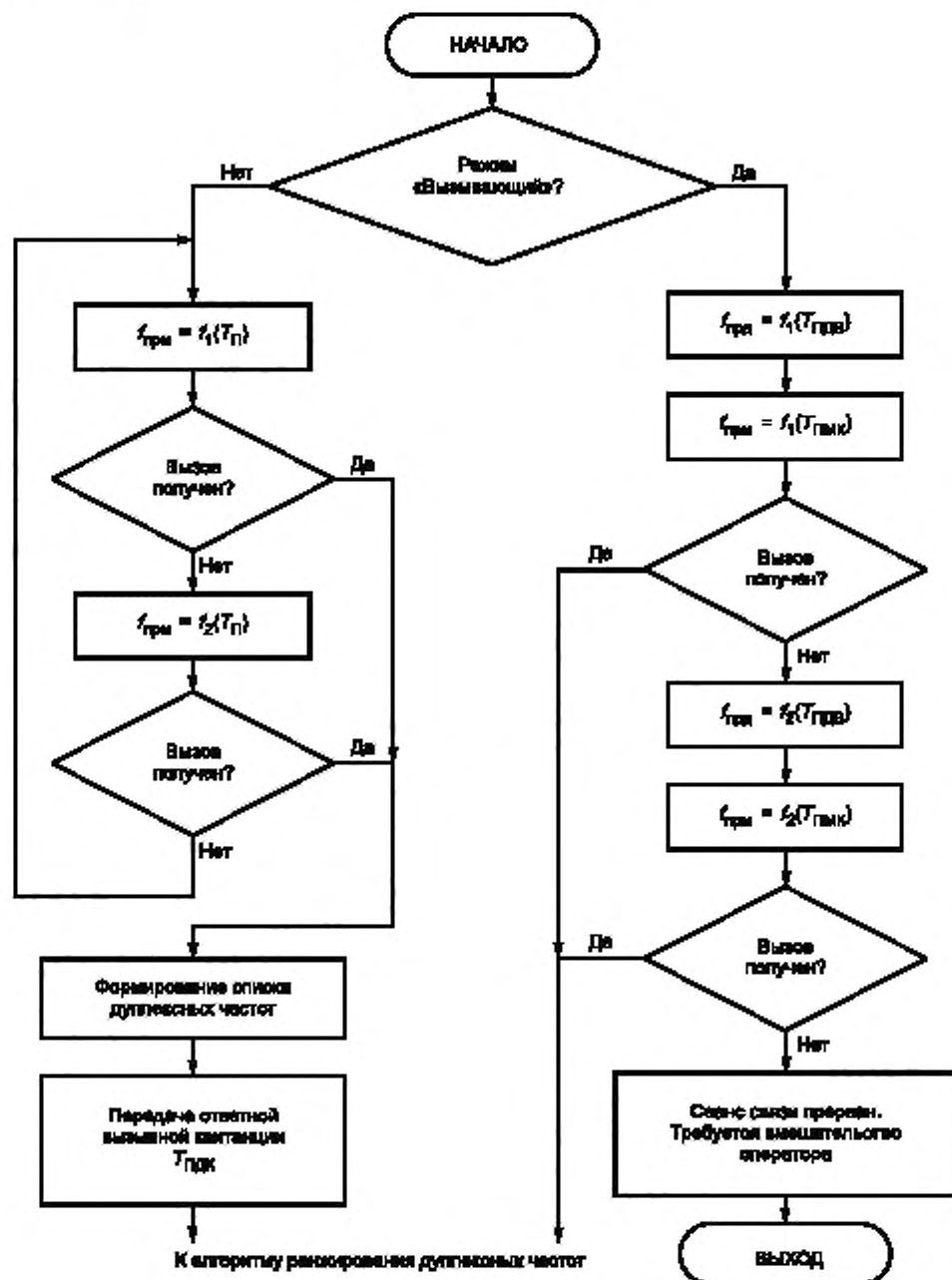
Рисунок 1 — Блок-схема алгоритма входящего вызова
