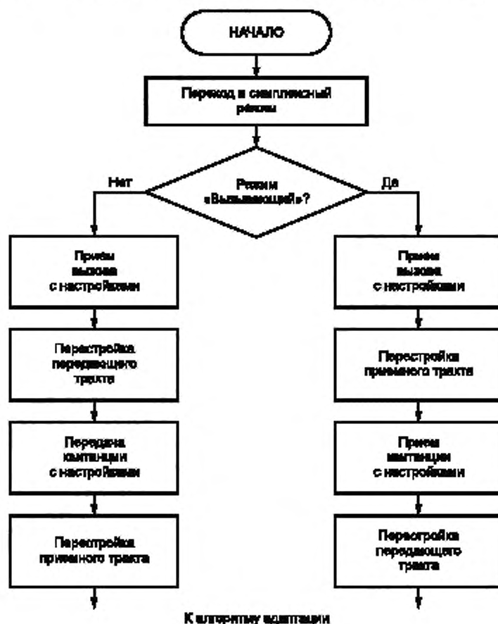
Рисунок 3 — Блок-схема алгоритма перехода в дуплексный режим
