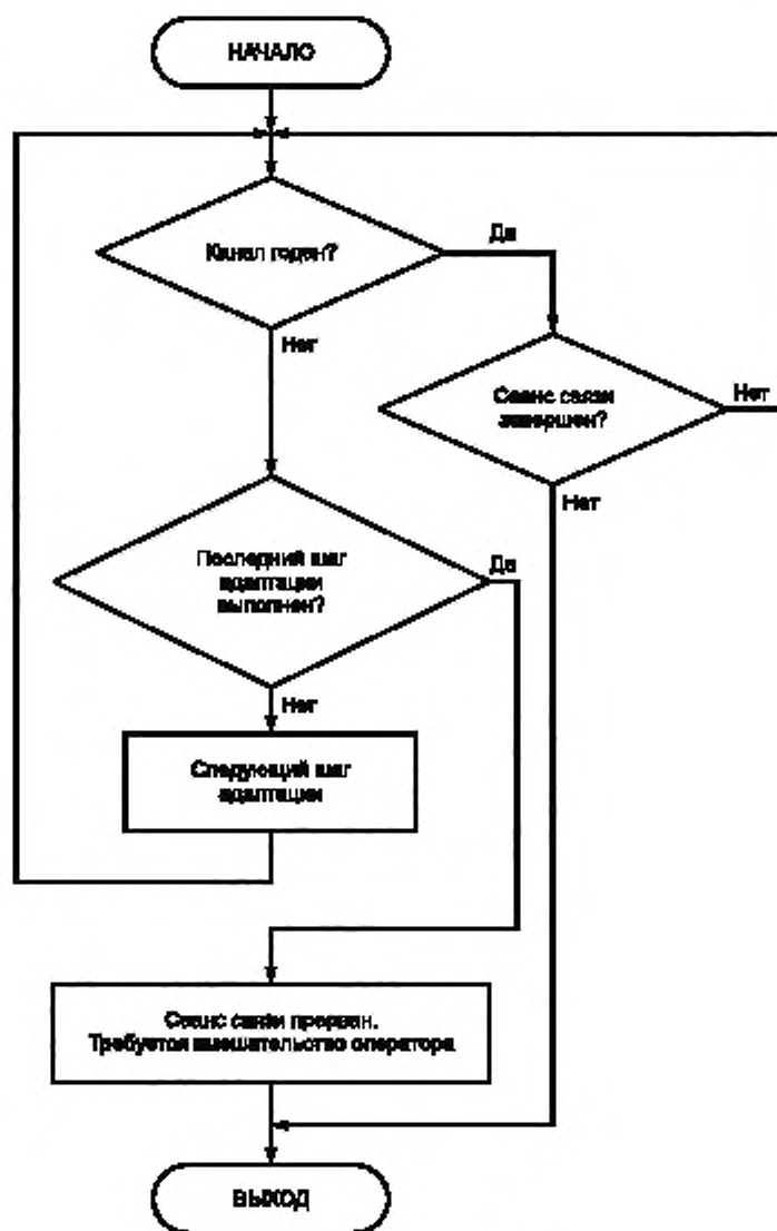
Рисунок 4 — Блок-схема алгоритма адаптации
