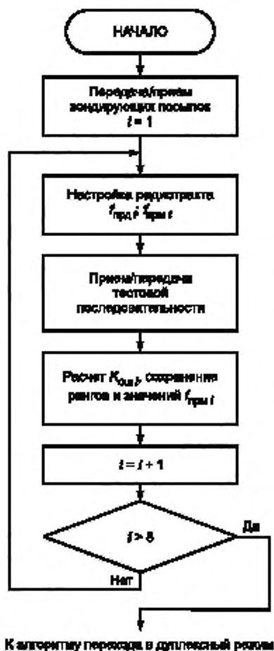
Рисунок 2 — Блок-схема алгоритма ранжирования частот радионаправления
