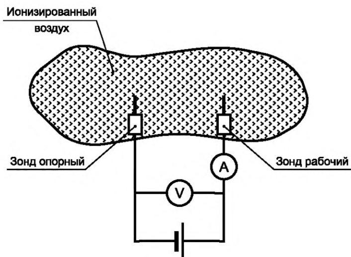
Рисунок 2 — Схема установки
