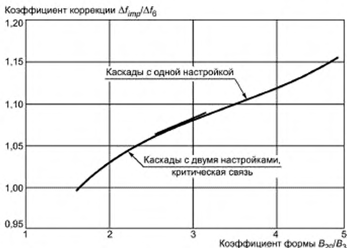
Рисунок Е.1 — Коэффициент коррекции для оценки отношения B_{imp}/B_0 для других типов настраиваемых схем
