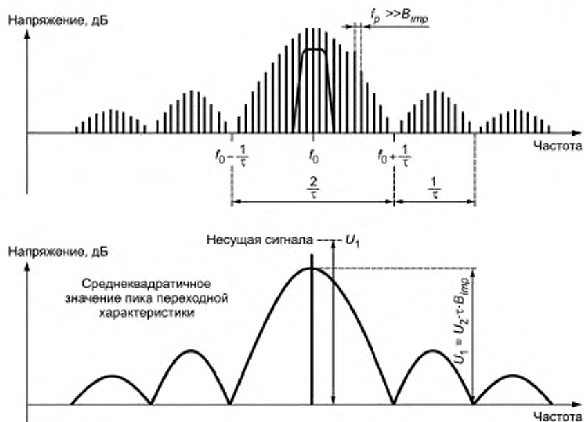
Рисунок E.6 — Фильтрация, когда значение B_{\text{имп}} намного больше частоты повторения импульсов
