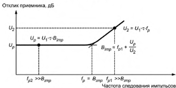
Рисунок E.7 — Расчет ширины импульсной полосы пропускания ИП
