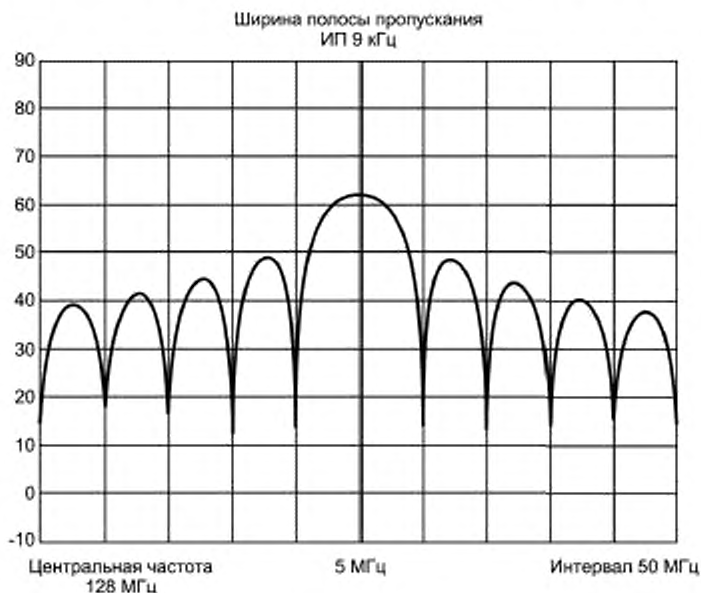
Рисунок Е.3 — Спектрограмма импульсно-модулированного сигнала при ширине импульсов 200 нс
