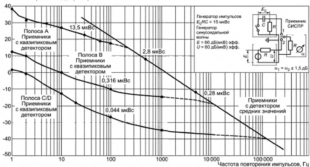
д) Теоретические кривые импульсной характеристики ИП с квазилинейным детектором и детектором средних значений (см. 6.4.2)
