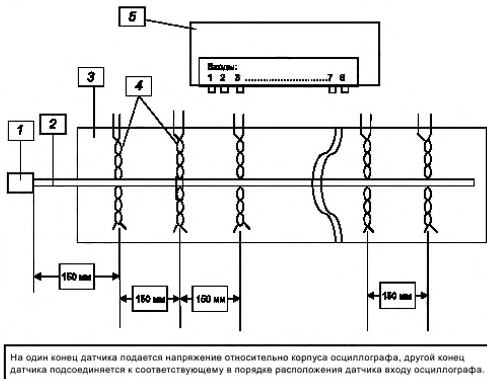
1 — электродетонатор; 2 — образец испытуемого шнура; 3 — основание; 4 — датчики; 5 — осциллограф
