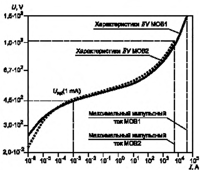
Рисунок Е.2 — Сравнение вольтамперных характеристик двух MOV
