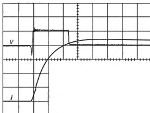
I Входной ток NID 50 A/div. dI/dt = 75 \text{ A}/\mu\text{s} V Напряжение между телефонным портом и защитным проводником (PE) 200 В/дел: максимум 200 В Горизонтальная развертка: 2 мкс/деление
