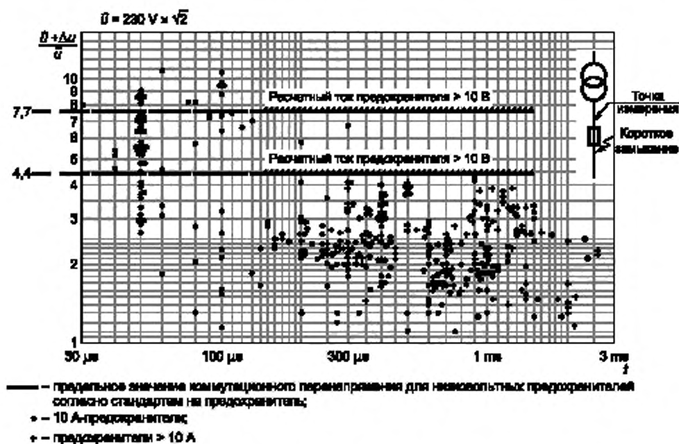
Рисунок В.11 — Зависимость перенапряжения от продолжительности коммутационных импульсных перенапряжений в системе электроснабжения. Короткое замыкание вблизи предохранителя отходящей линии
