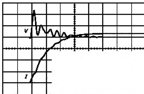
I Входной ток NID 50 A/div; dI/dt = 75 A/мкс V Напряжение между телефонным портом и защитным проводником (PE) 2 кВ/дел; максимум 4,3 кВ. Горизонтальная развертка: 2 мкс/дел
