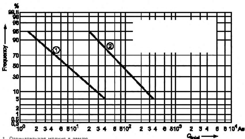
Рисунок А.2 — Частотное распределение полного заряда молнии Q_{\text{total}}
