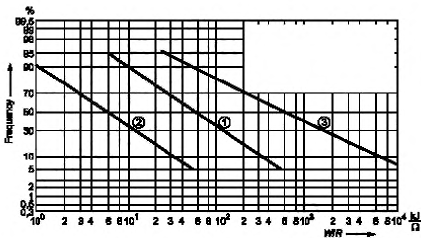
Рисунок А.3 — Частотное распределение переходного заряда молнии Q_{\text{транс}}
