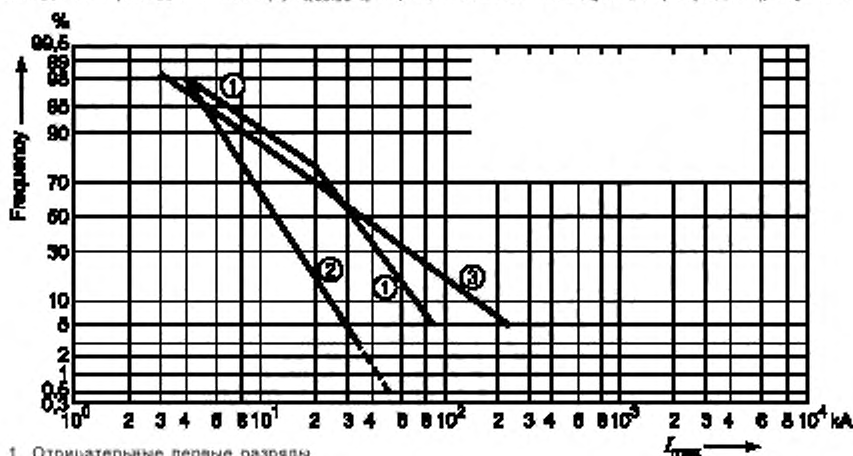
Рисунок А.1 — Частотное распределение максимального тока молнии I_{\max}
