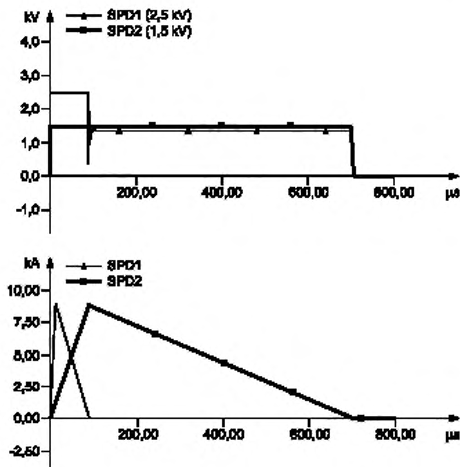
Рисунок E.7 — Расчетные напряжение и ток УЗИП для импульса тока 10/350 мкс, введенного в узле 2
