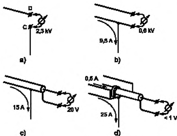
Рисунок F.3 — Измерение напряжения в диспетчерской на кабеле, замкнутом на первичной стороне трансформатора. Токи обычного вида для различных параллельных заземляющих проводников между точками A и C.
