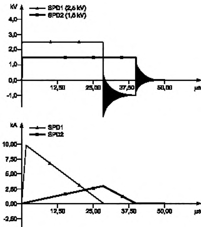
Рисунок E.6 — Расчетные напряжение и ток УЗИП для импульса тока 2/20 мкс, введенного в узле 1
