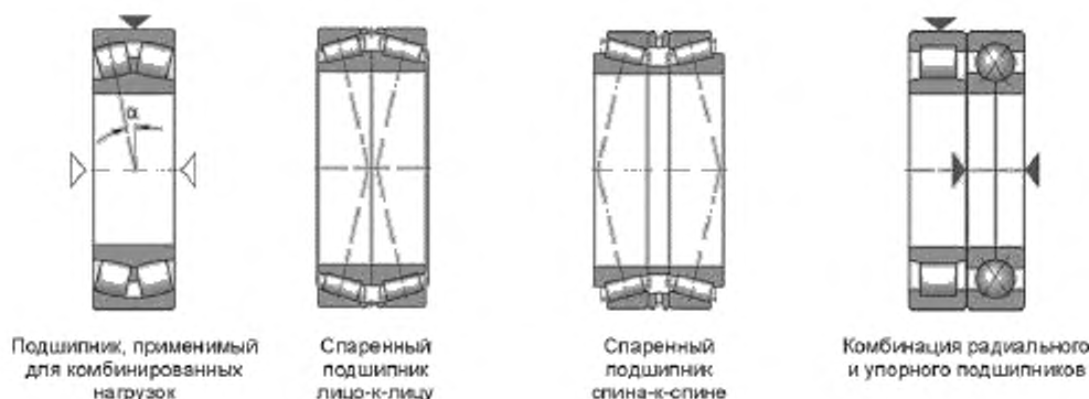
Рисунок 26 — Примеры расположений упорных подшипников
