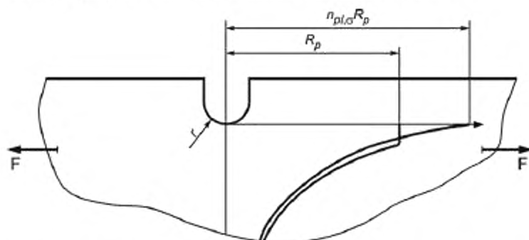
Рисунок 7 — Определение параметра сечения n_{pl,\sigma} компонента с пазом
