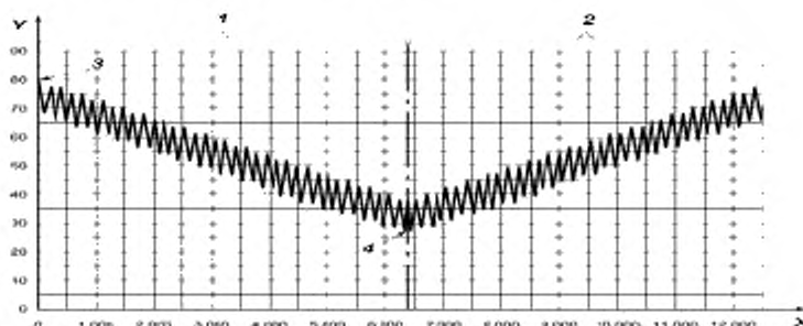
X – время, с; Y – SOC, %; 1 – постепенный циклический разряд; 2 – постепенная циклическая зарядка; 3 – начальная SOC = 80 %; 4 – поворотная точка цикла при SOC = 30 % (примечание – достижение SOC = 30 % является поворотной точкой цикла)
