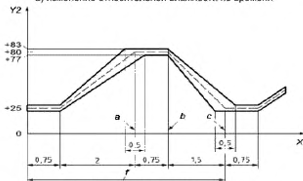
б) изменение температуры по времени
