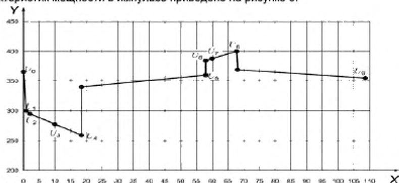
Рисунок 6 — Снятие характеристик мощности в импульсе (график по напряжению).
