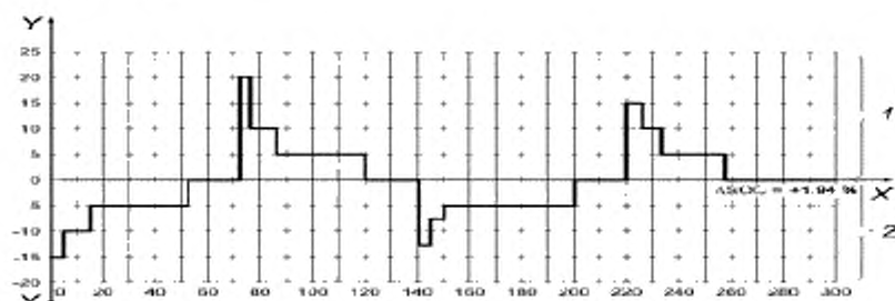
X – время, с; Y – ток (в величинах, кратных C): 1 – разряд; 2 – зарядка.
