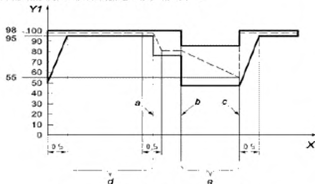
а) изменение относительной влажности по времени
