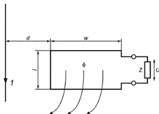
Рисунок G.2 — Механизм магнитного взаимодействия
