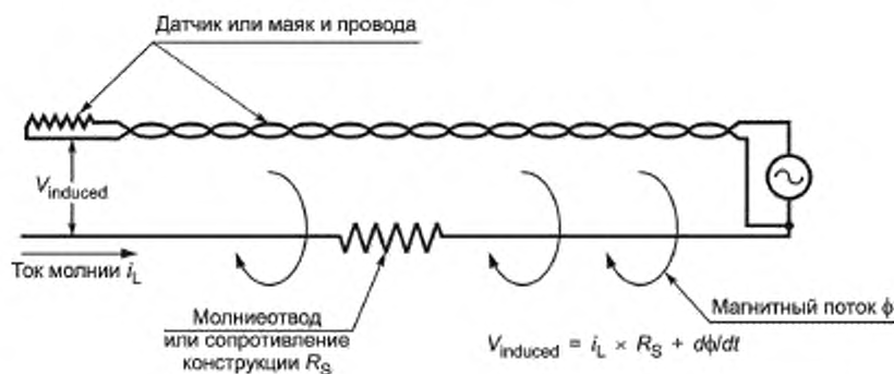
Рисунок С.3 — Индуцированные молнией напряжения между молниеотводом или конструкцией и проводами датчика
