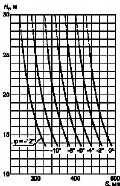
Рисунок А.23 — Графики линий равных углов в координатах H_t - S
