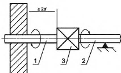
d – наружный диаметр; 1, 2 – труба; 3 – испытуемый образец
