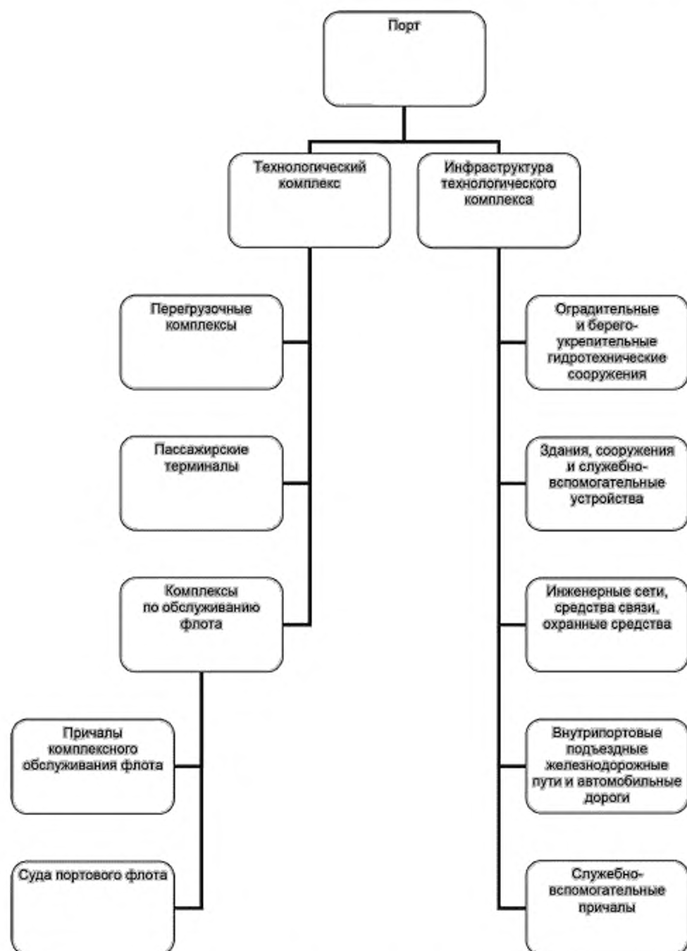
Рисунок А.3 — Функциональная схема речного порта
