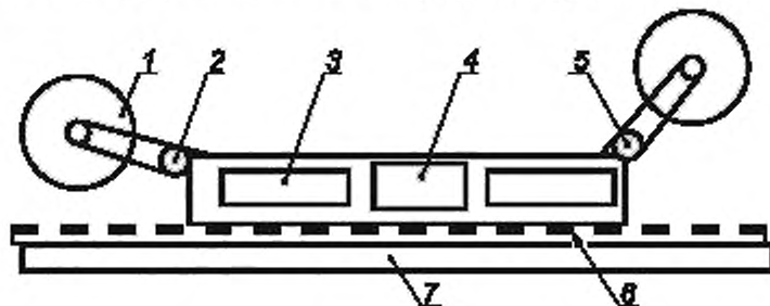
1 — шнек с резаками; 2 — поворотный редуктор; 3 — отделение редуктора; 4 — распределительное устройство; 5 — электродвигатель привода шнека; 6 — расположение реечной передачи; 7 — забойный скребковый конвейер
