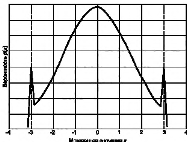
Рисунок А.3 — Негавуссовская плотность вероятности распределения
