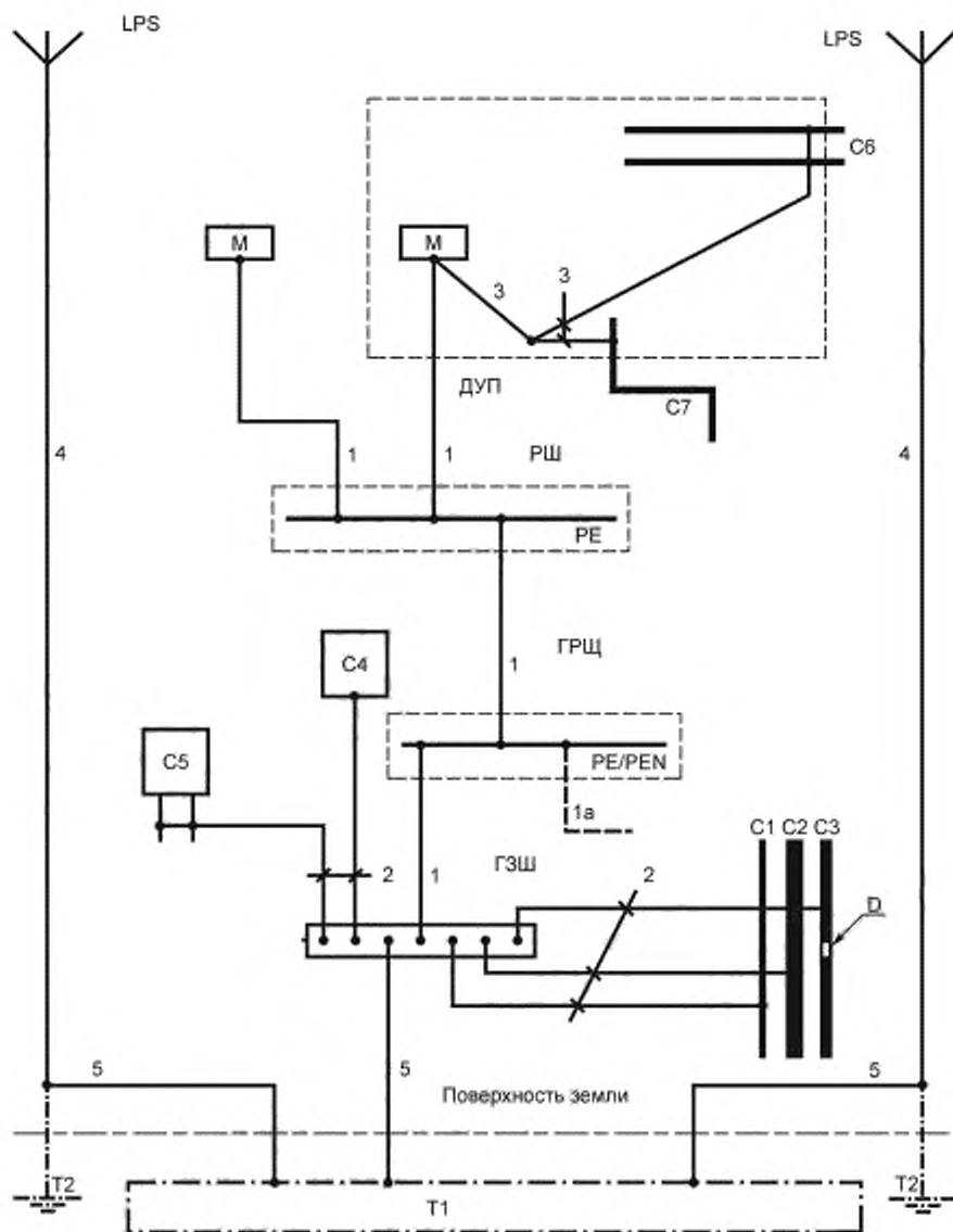
Пример размещения заземляющего устройства и защитных проводников
