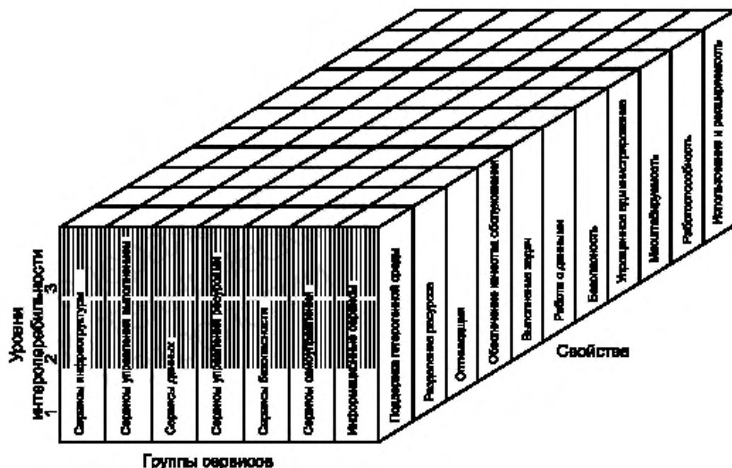
Рисунок 2 — Модель СОАОГС
