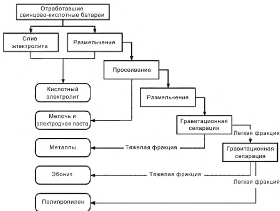
Рисунок 2 — Процесс разделки отработавших свинцово-кислотных батарей
