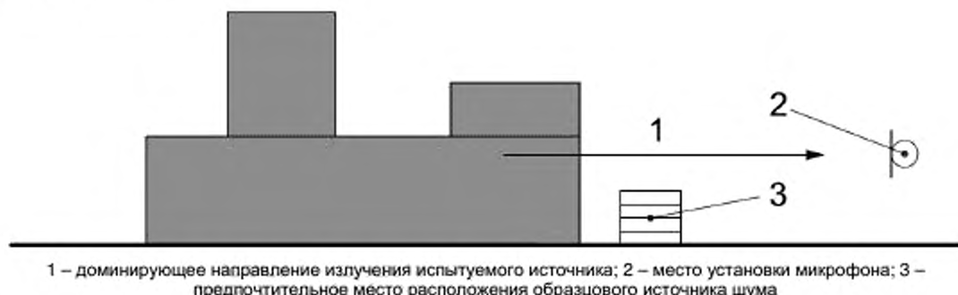
Рисунок В.2 – Место расположения образцового источника шума в случае испытуемого источника с доминирующим направлением излучения
