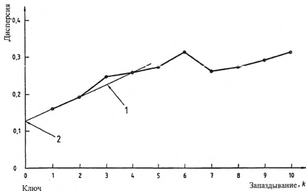
Рисунок 3 Вариограмма для данных из таблицы А.2
