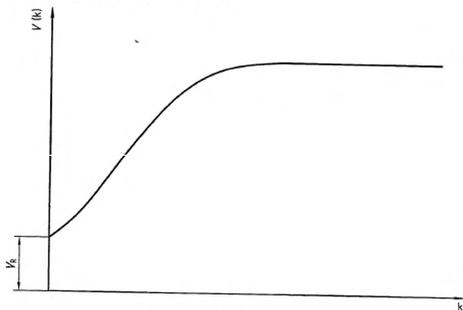
Рисунок A.2 – Общий вид вариограммы
