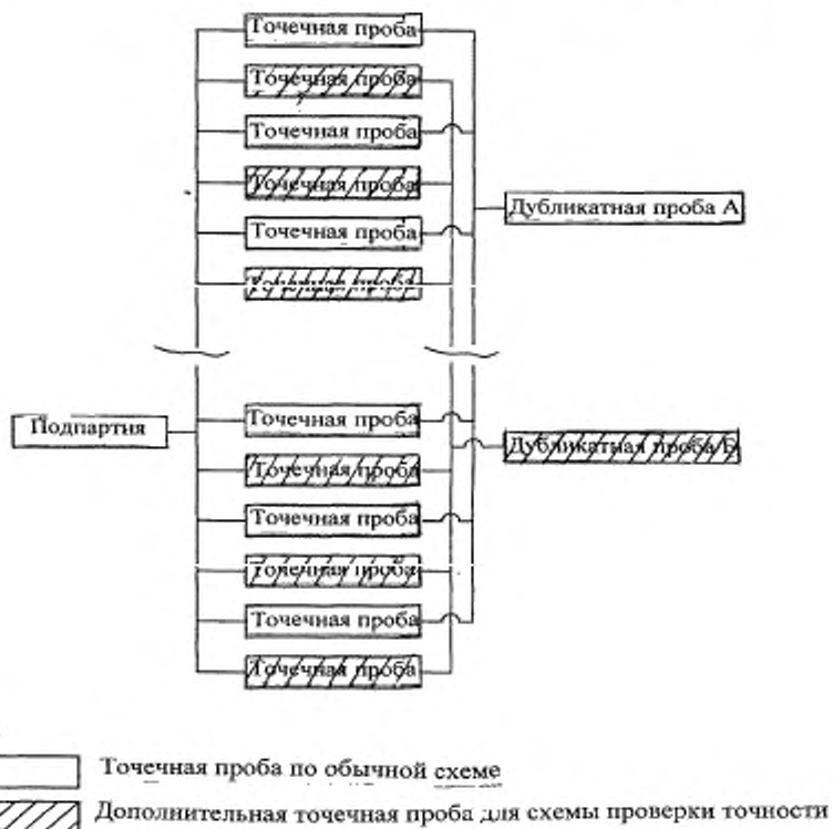
Рисунок 1. Пример плана дубликатного опробования
