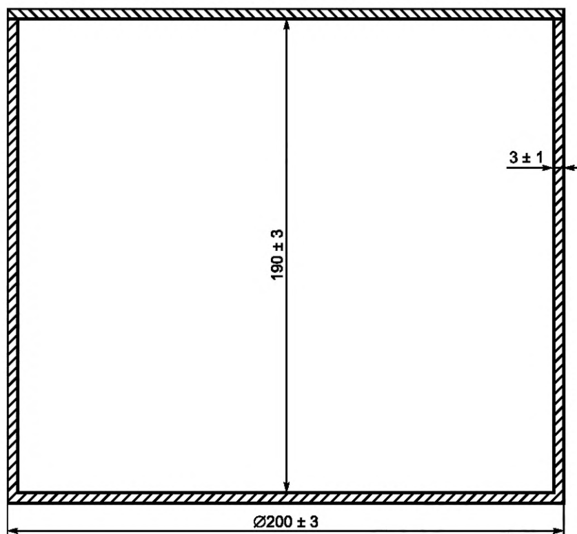
Рисунок 2 — Цилиндрический фантом головы
