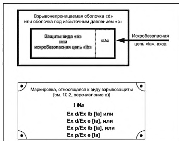
Рисунок 4 — Оборудование уровня взрывозащиты Ma (защита вида «e» или искробезопасная цель «ib» внутри взрывонепроницаемой оболочки «d» или оболочки под избыточным давлением «p»)
