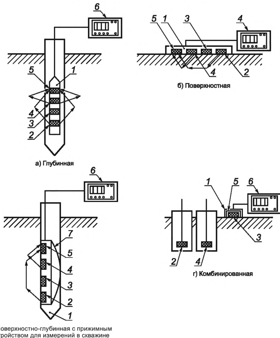
Рисунок 4 — Схемы измерений радиоизотопными влагоплотномерами
