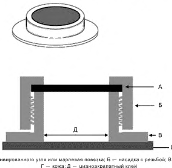
Рисунок 1 — Пример стандартного устройства, используемого для ограничения и защиты места нанесения вещества во время исследований перкутанной абсорбции in vivo
