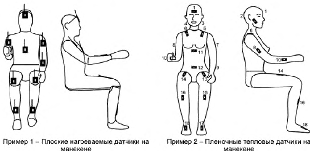
Рисунок А.2 – Примеры установки датчиков для измерения t_{\text{eq}} с использованием нескольких отдельных нагреваемых датчиков, прикрепленных к манекену или реальному человеку
