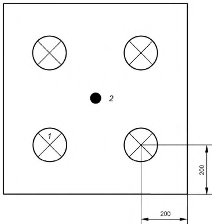
Рисунок 3 — Схема размещения растений и тензиометра в питательном грунте испытательного контейнера размерами 800 × 800 мм
