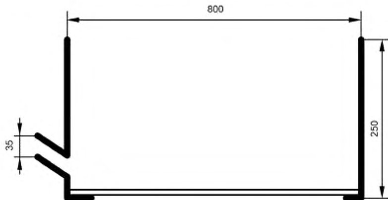
Рисунок 1 — Конструкция контейнера
