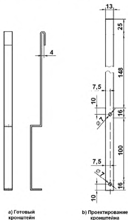
Рисунок 2 — Держатель для термометра
