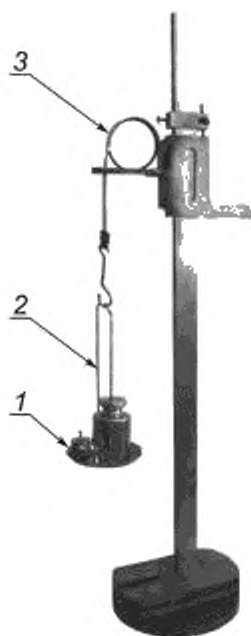
1 — чашка с гирьками; 2 — подвеска; 3 — поршневое кольцо с незамкнутым замком
