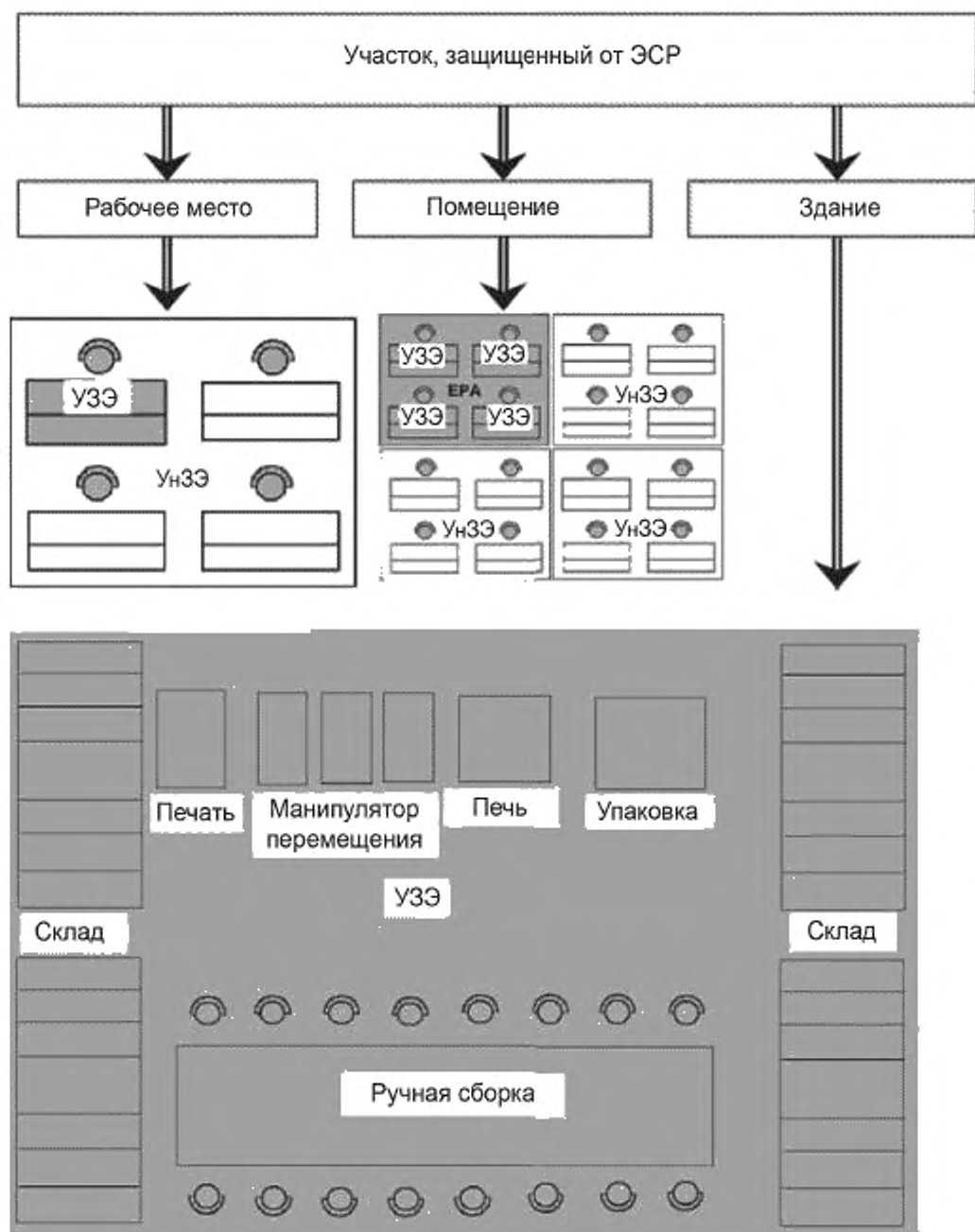
Рисунок 2 — Пример схемы УЗЭ
