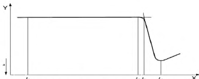
Рисунок 4 — Типичная кривая ДСК при определении термостабильности
