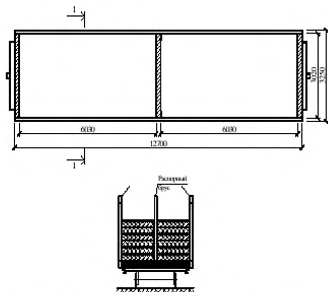
Рисунок 4 – Схема контейнера для перевозки плит
