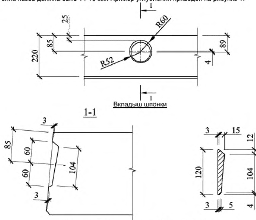
Рисунок 1 – Углубление на боковой поверхности плиты
