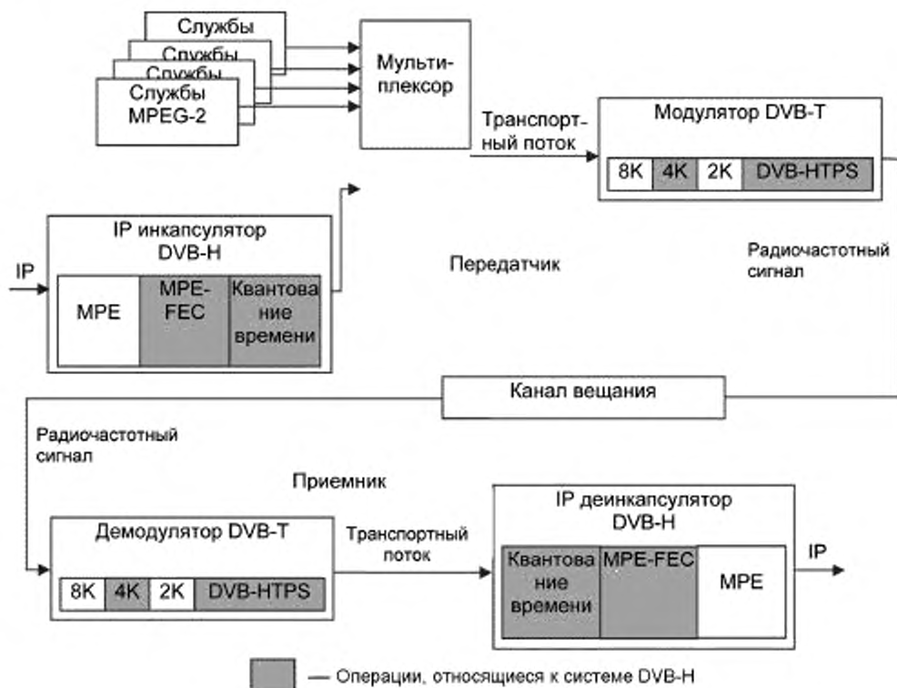
Рисунок 2 — Концептуальная структура системы DVB-H
