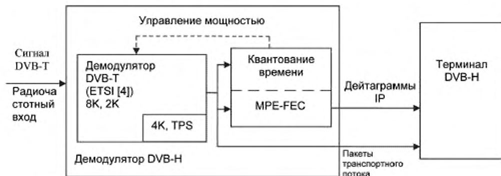
Рисунок 1 — Концептуальная структура приемника DVB-H
