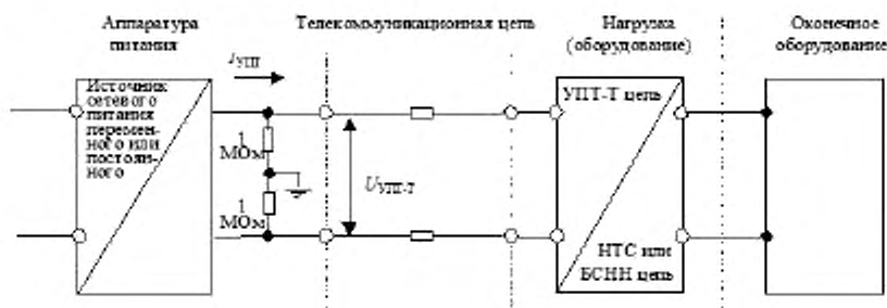
Рисунок А.1 – Пример УПТ-Т системы удаленного электропитания
