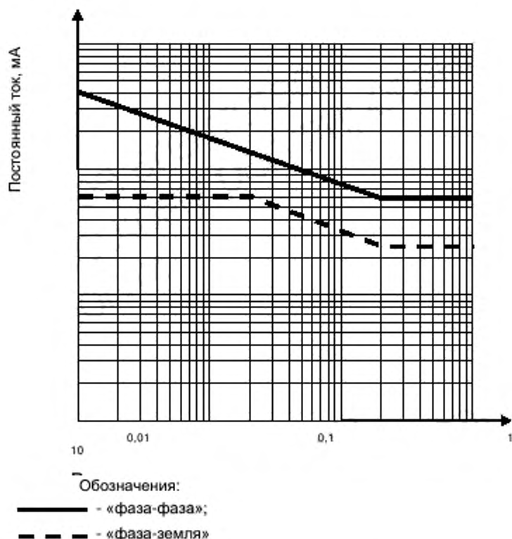
Рисунок 1 – Максимальный ток после единичной неисправности
