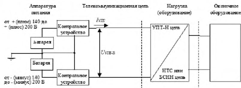
Рисунок 2 – Пример УПТ-Н системы удаленного электропитания
