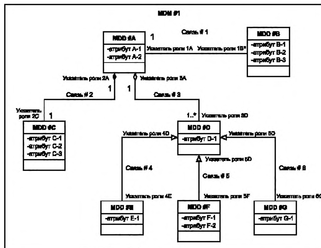
Рисунок 4 — Пример структуры MDM-модели
