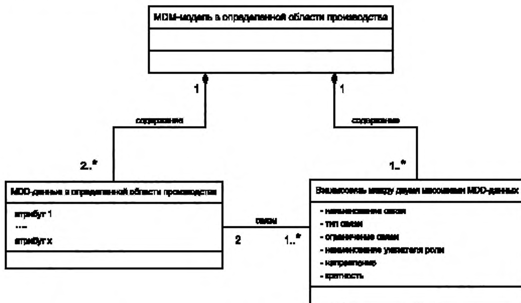
Рисунок 5 — Блок-схема, иллюстрирующая взаимосвязи между MDD-данными и MDM-моделью
